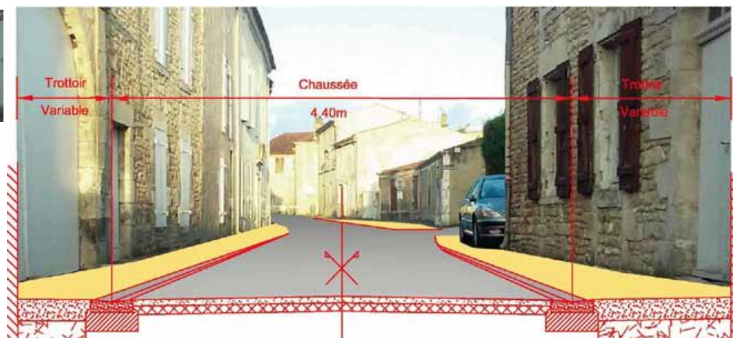
Profil de la rue de la République (avant / après)
