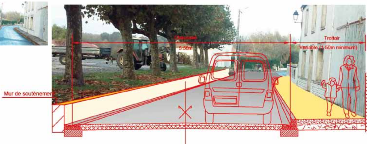
Profil de la rue du 19 mars (avant / après)
